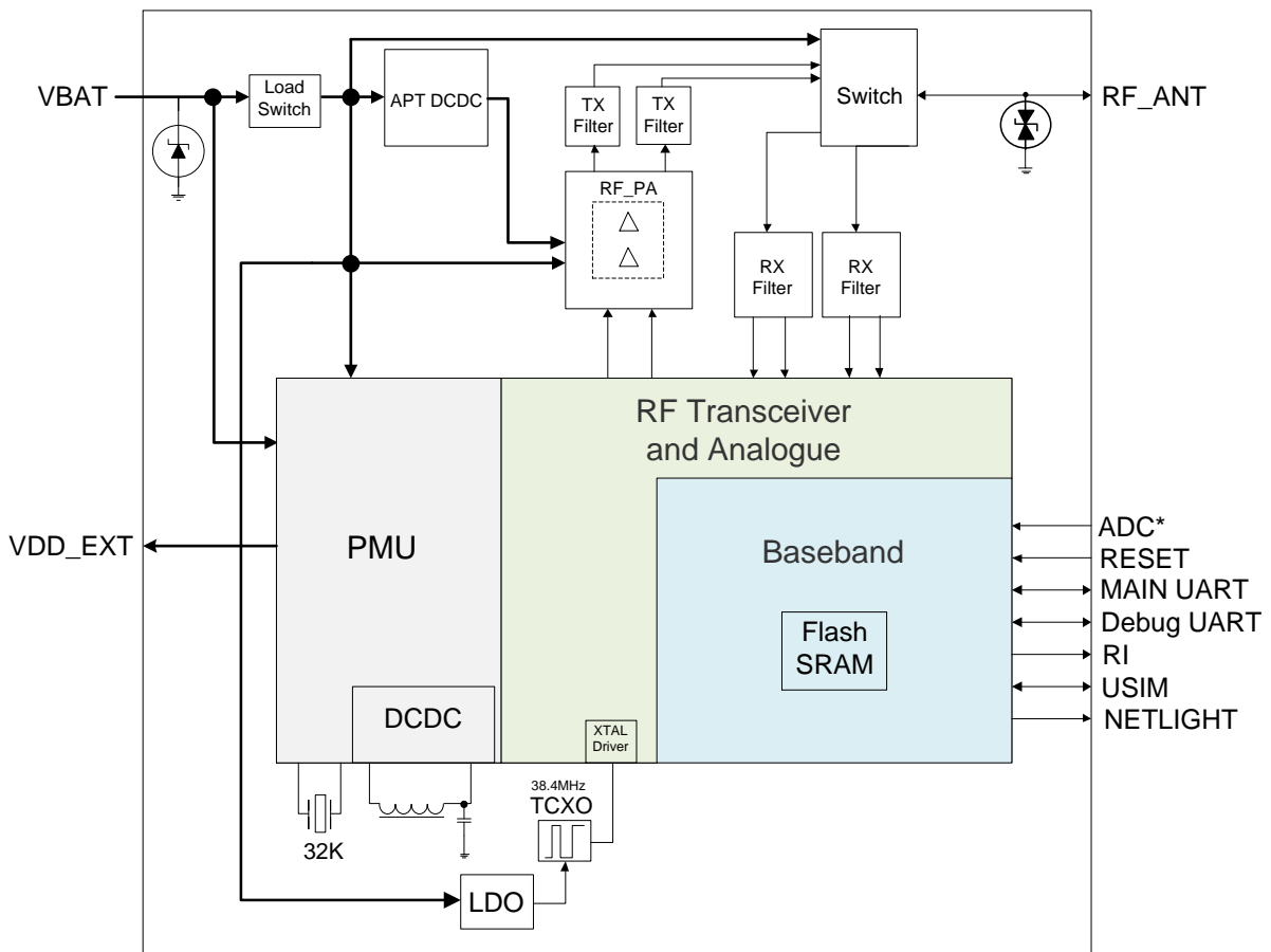
图 1：功能框图
