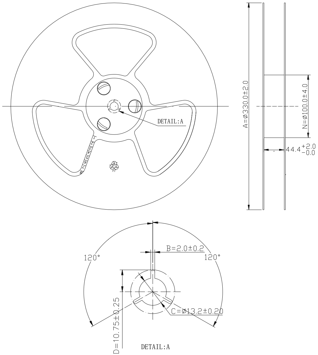
图 31: 卷盘尺寸 (单位: 毫米)
