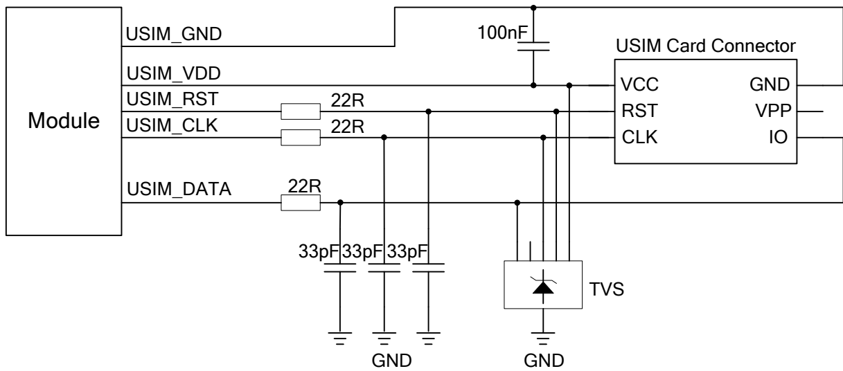
图 13: 6-pin 外部 USIM 卡座参考电路图
