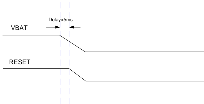
图 6：关机时序
