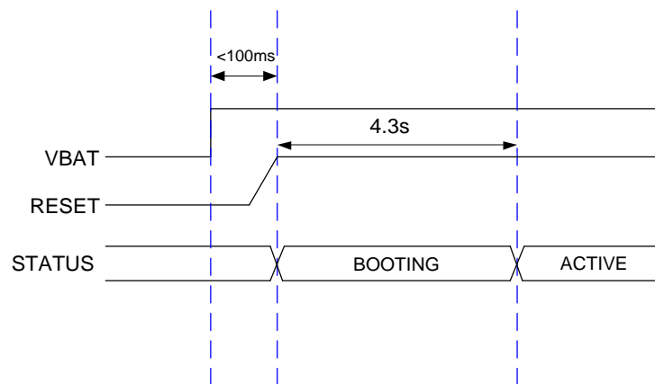
图 5: 开机时序
