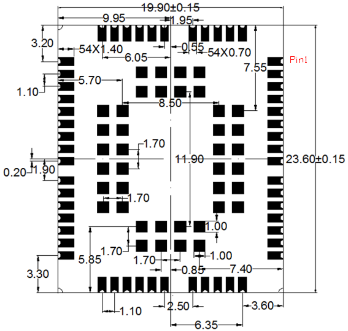
图 25: 底视尺寸图
