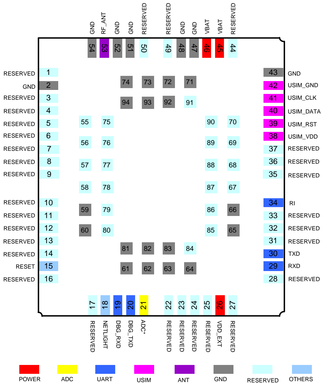
图 2: 引脚分配图
