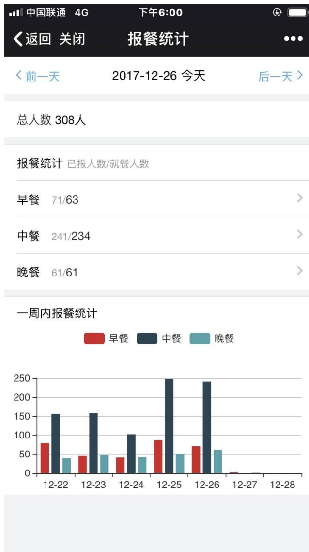
微信端统计
